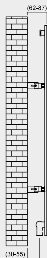
BOČNÍ POHLED
